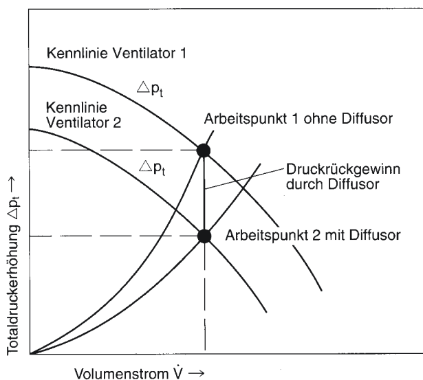
Bild 2: Druckrückgewinnung
