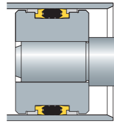
Пример монтажа
