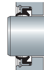
Пример монтажа SCB
