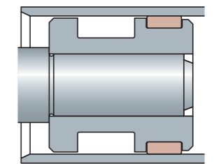
Пример монтажа для поршней
