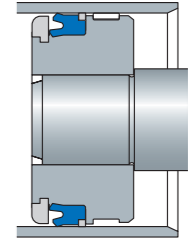
Пример монтажа
