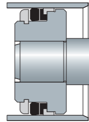
Пример монтажа
