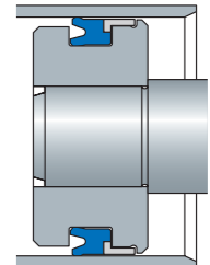
Пример монтажа
