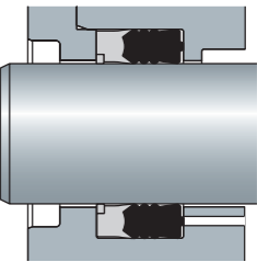
Пример монтажа
