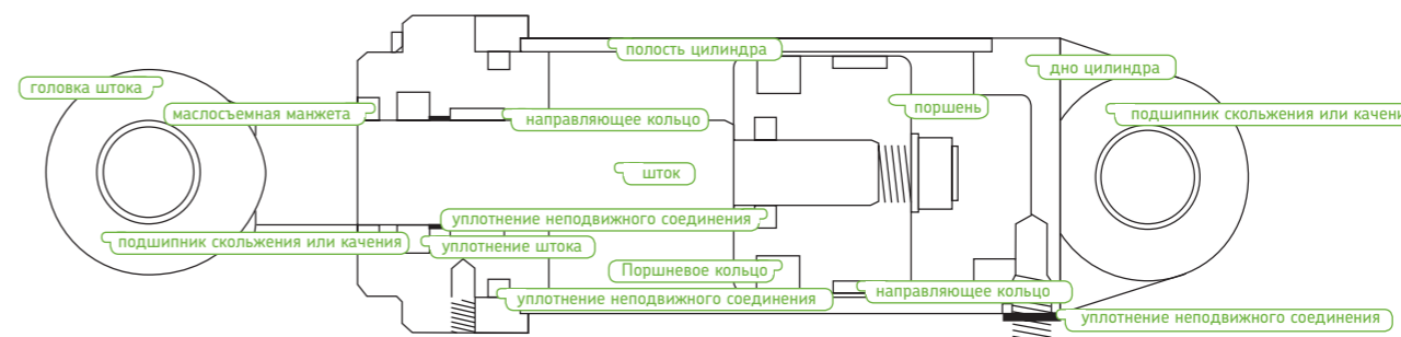
Гидравлический цилиндр – Терминология
