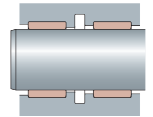
Пример монтажа для штоков
