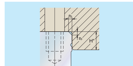
Fig. 6 Ball slide datum face
